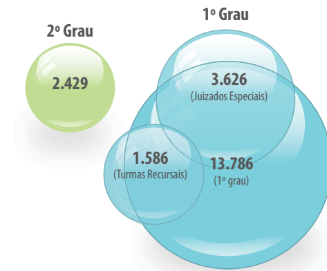
Figura 3: Exemplo de uso do Diagrama de Venn
